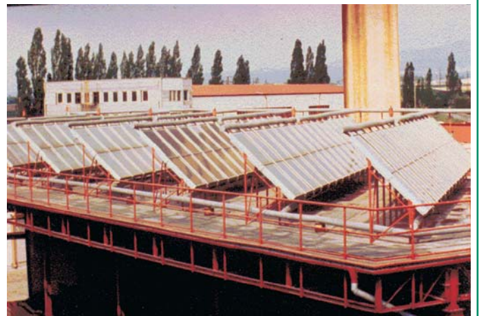
▲ Solárny ohrev teplej úžitkovej vody 14500 l/deň Typ slnečného kolektora: Salk 200 1.V Počet slnečných kolektorov: 100 ks Absorbčná plocha kol. poľa: 200 m 2 Energetický zisk kol. poľa: 120.200 kWh/rok
